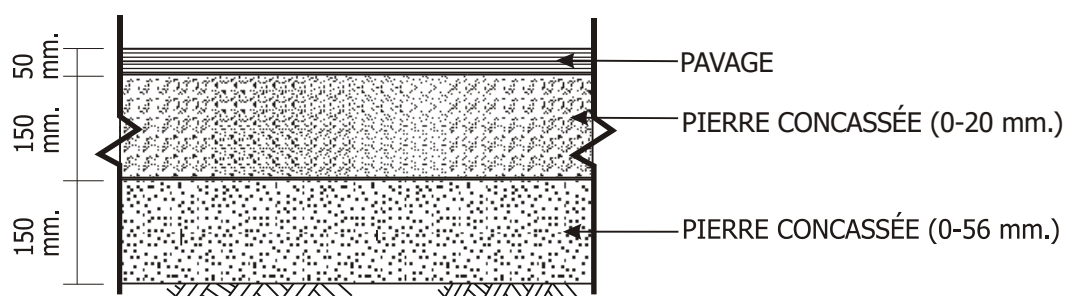
Figure 2 : Pavage et fondation – Coupe type
